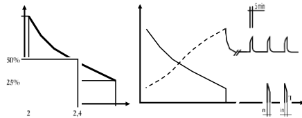
Curva di carica di tipo "wa" (din 41774) "Wa" characteristic (din 41774)
